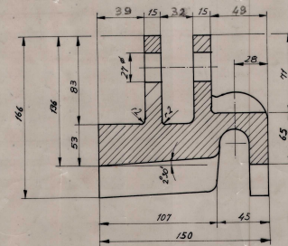
A-A KESİTİ
